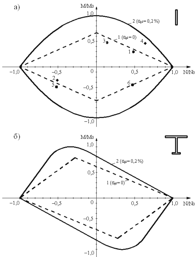
Рис. 6. Области относительной прочности для прямоугольного (а) и двугаврового (б) сечений при \varepsilon_{pl} = 0 (линия 1) и \varepsilon_{pl} = 0,2\% (линия 2)
